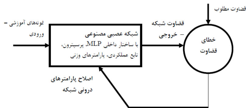
شکل(۱): نمایی از نحوی آموزش یک شبکه عصبی
