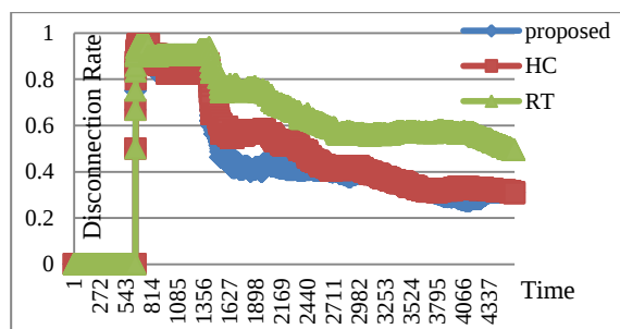
شکل ۱۱: نرخ قطع شدن سرویس در سناریوی ۵
