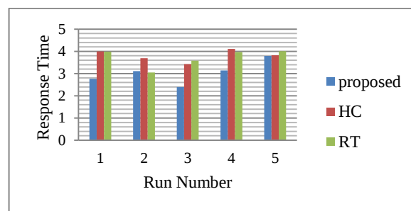
شکل ۸: زمان پاسخ سرویس دهندگان در سناریوی ۳
