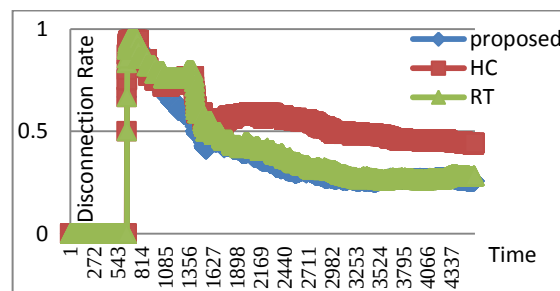
شکل ۹: نرخ قطع شدن سرویس در سناریوی ۴
