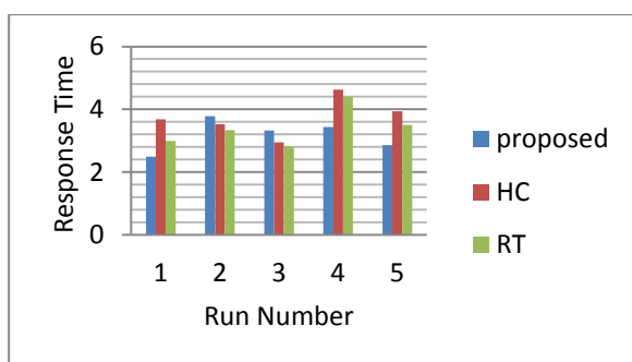
شکل ۴: زمان پاسخ سرویس دهندگان در سناریوی ۱
