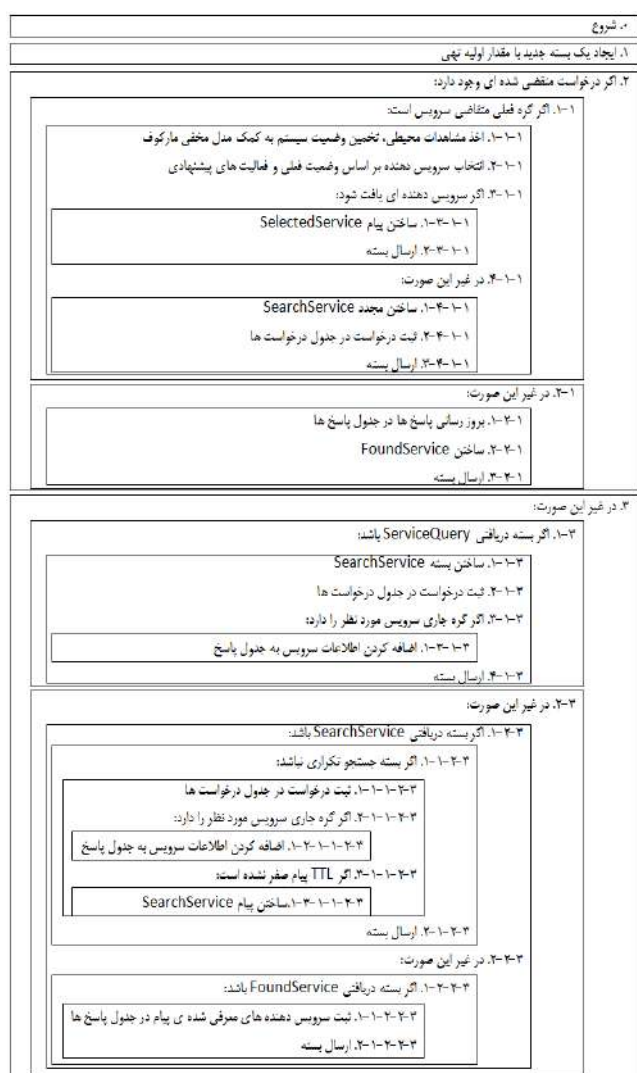
شکل ۲: الگوریتم پیشنهادی
